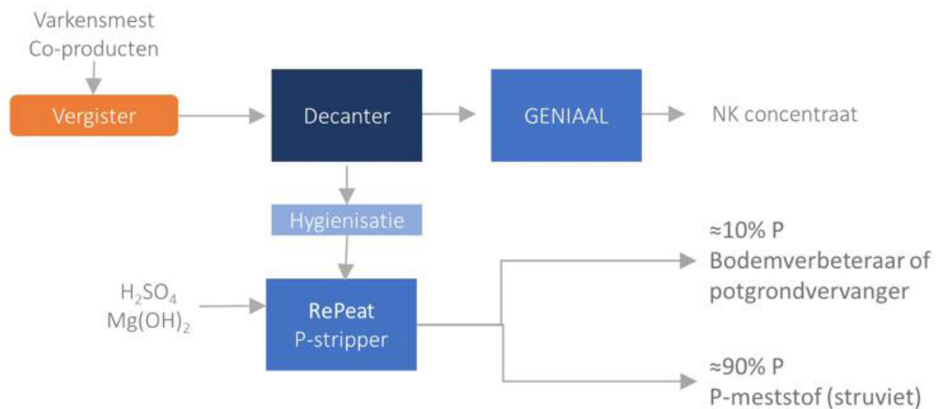
Figuur 3. De verwerking van (varkens)drijfmest in de Groene Mineralen Centrale bij Groot Zevert Vergisting. Bron: https://www.groenemineralencentrale.nl/nl/re-p-eat
