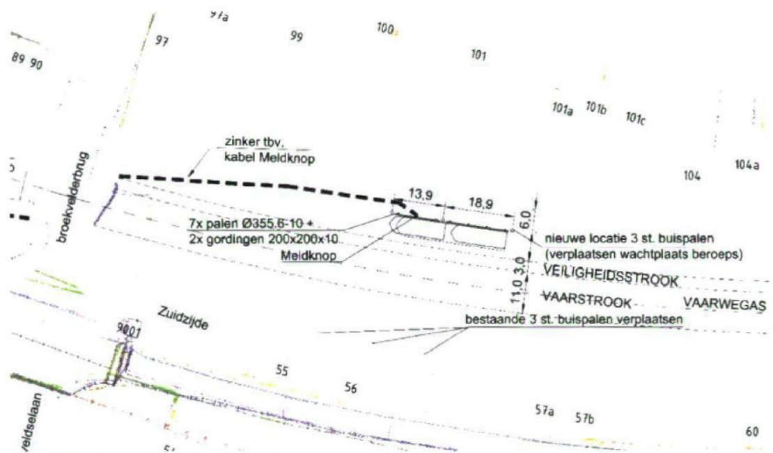
Afb. 1 Ontwerptekening wachtplaats
