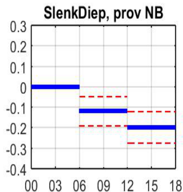
Figuur 3.3: Daling in stijghoogte Slenk\Diep
