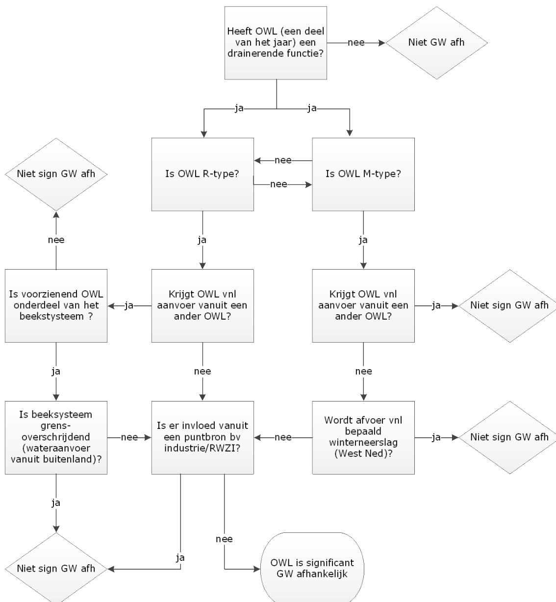
Fig 4.1. Stroomschema beoordeling wanneer oppervlaktewaterlichaam significant afhankelijk is van grondwater
