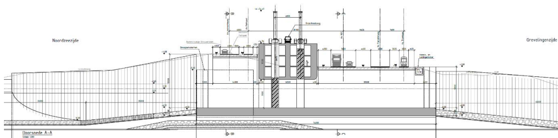
Figuur 8 dwarsdoorsnede doorlaatmiddel TF-VKA
