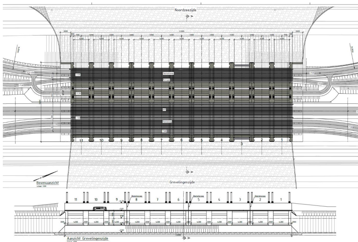
Figuur 9 bovenaanzicht en vooraanzicht doorlaatmiddel TF-VKA
