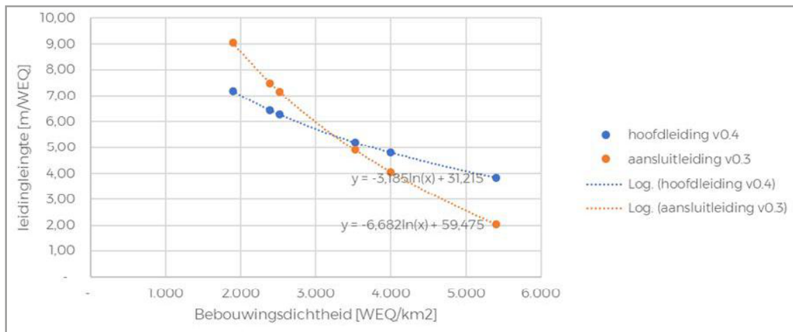
Figuur 22. Trendlijn hoofdleiding en aansluitleiding op basis van bebouwingsdichtheid
