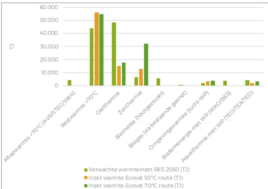
Figuur 31. Inzet warmtebronnen RES en Ecovatt routes (TJ)
