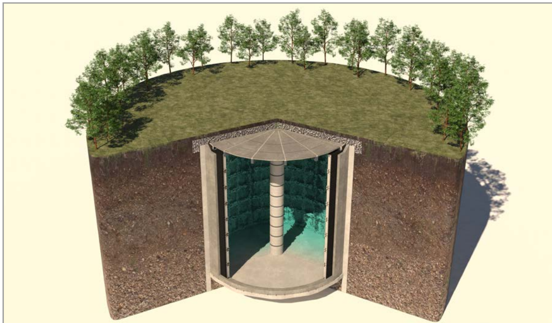
Figuur 4. Ecovat buffer
