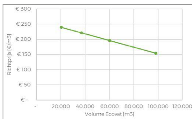
Figuur 24. Richtprijs Ecovat
