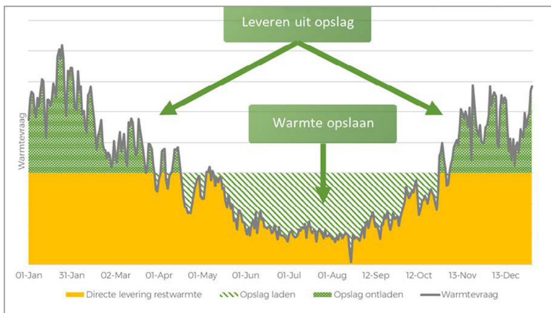
Figuur 9. Voorbeeldinvulling van de warmtevraag met restwarmte en warmteopslag
