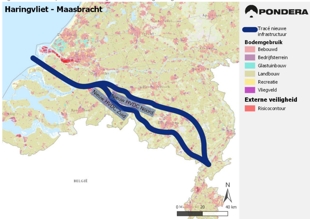
Figuur 43.1 - Tracéopties voor de ondergrondse verbinding Haringvliet–Maasbracht
