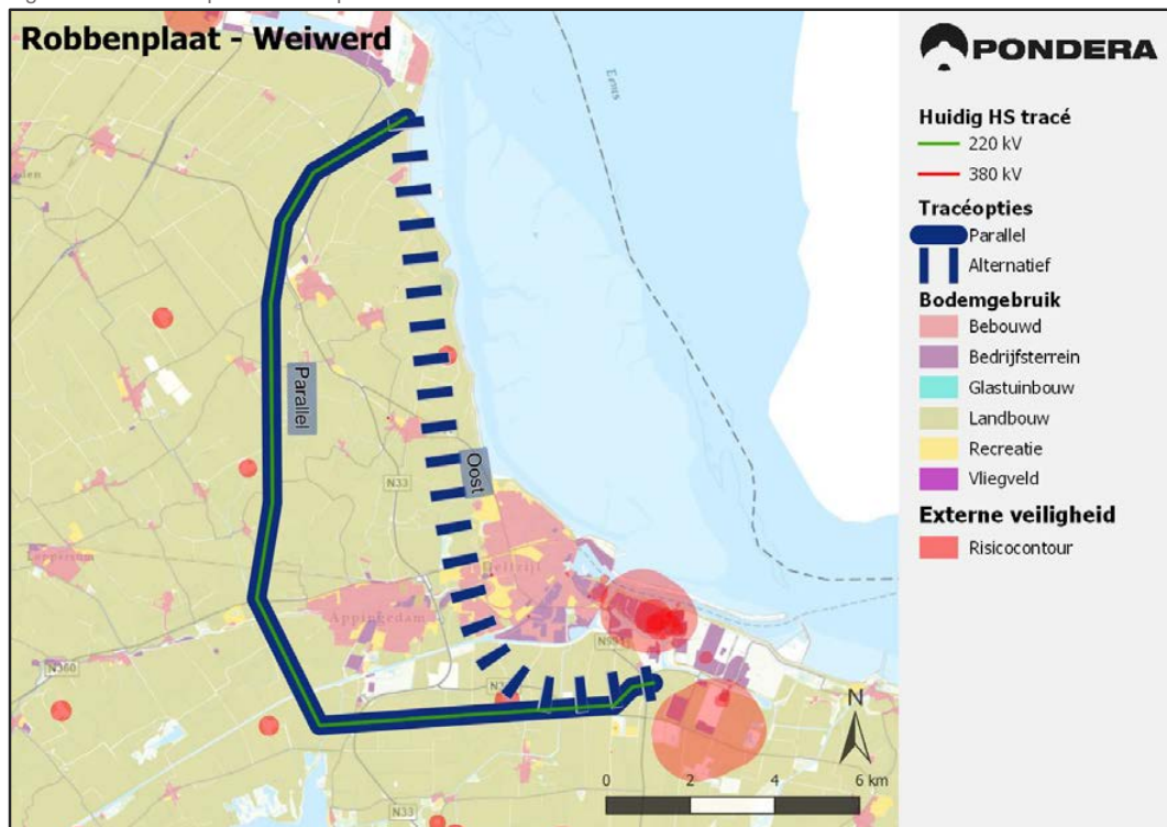
Figuur 38.1 - Tracéopties Robbenplaat–Weiwerd 220kV
