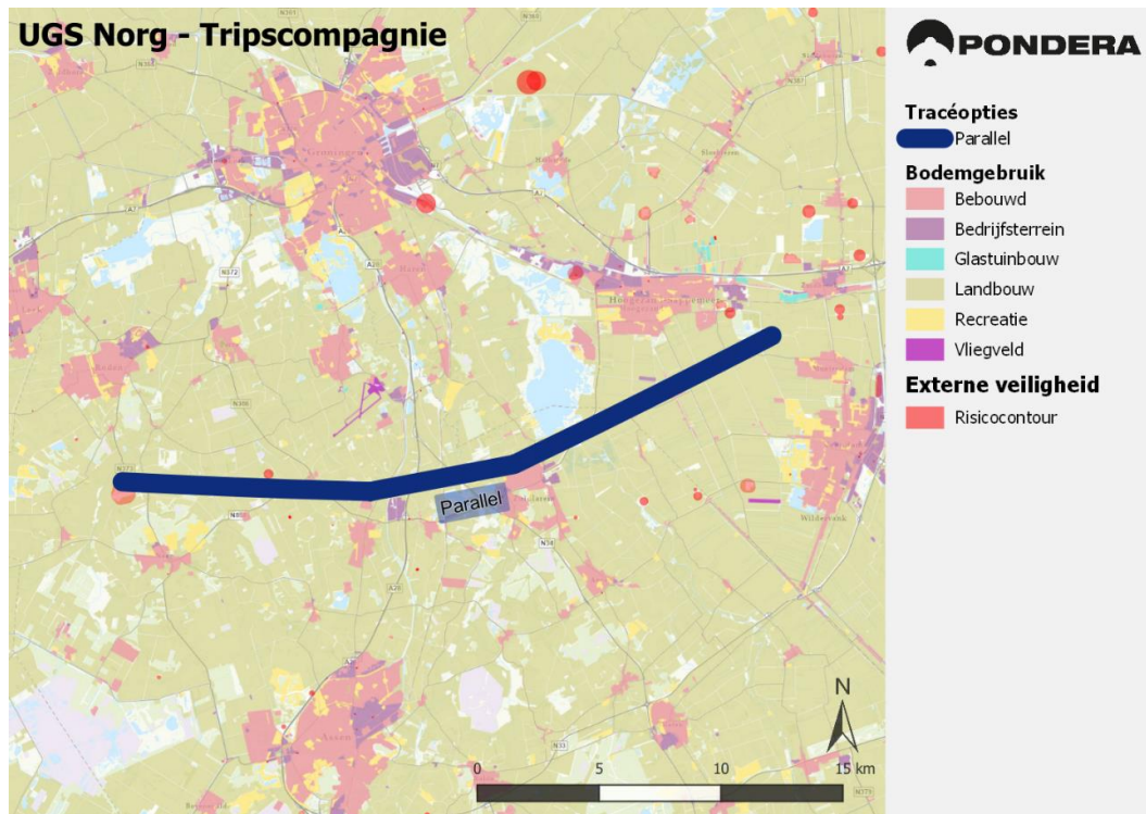
Figuur 3.4 - Tracéoptie UGS Norg – Tripscompagnie
