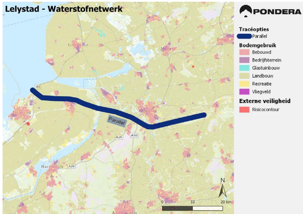
Figuur 3-3 - Tracéoptie Lelystad – Waterstofnetwerk
