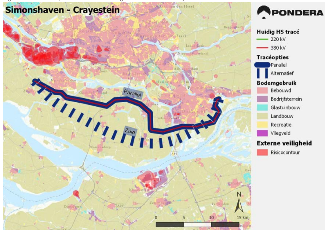
Figuur 39.1 - Tracéopties voor de verbindingen Simonshaven–Crayestein
