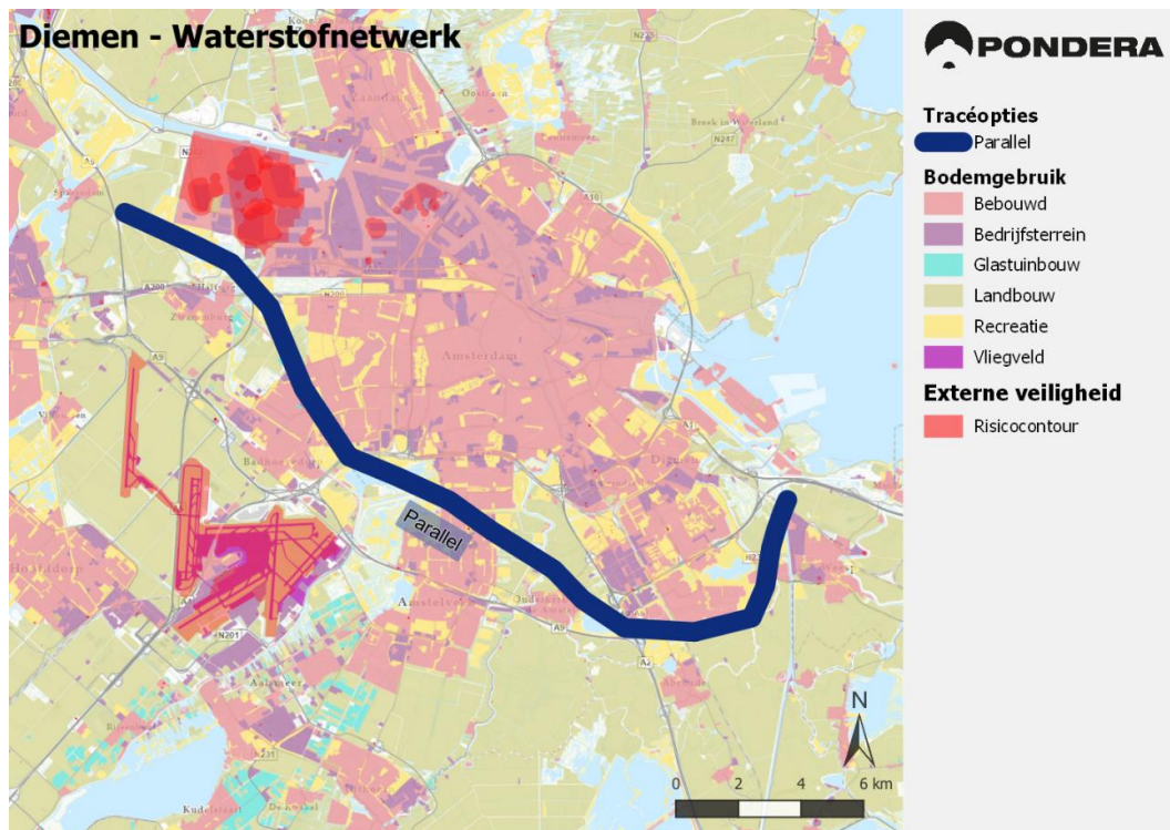
Figuur 3-2 - Tracéoptie Diemen-Waterstofnetwerk
