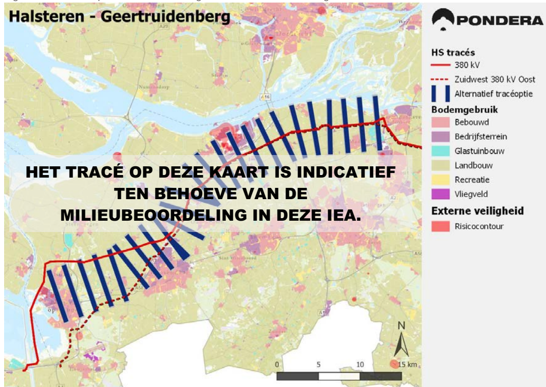
Figuur 31.1 - Tracéoptie voor de verbinding Halsteren–Geertruidenberg
