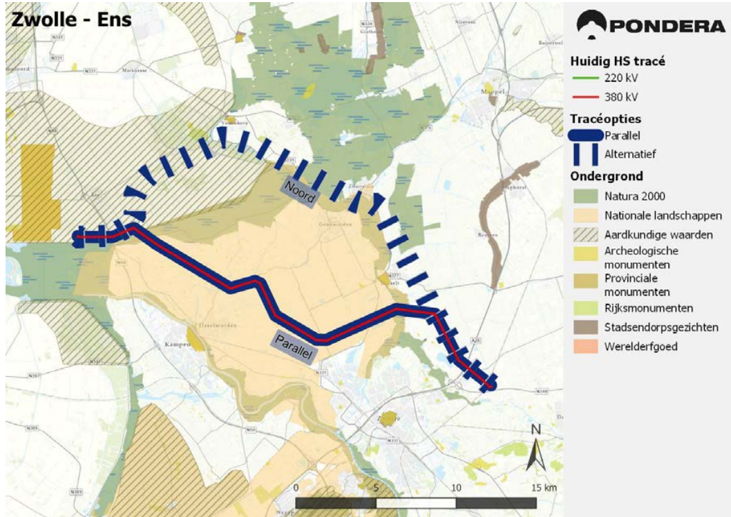
Figuur 2-3 - Tracéopties Zwolle-Ens ondergrondlaag
