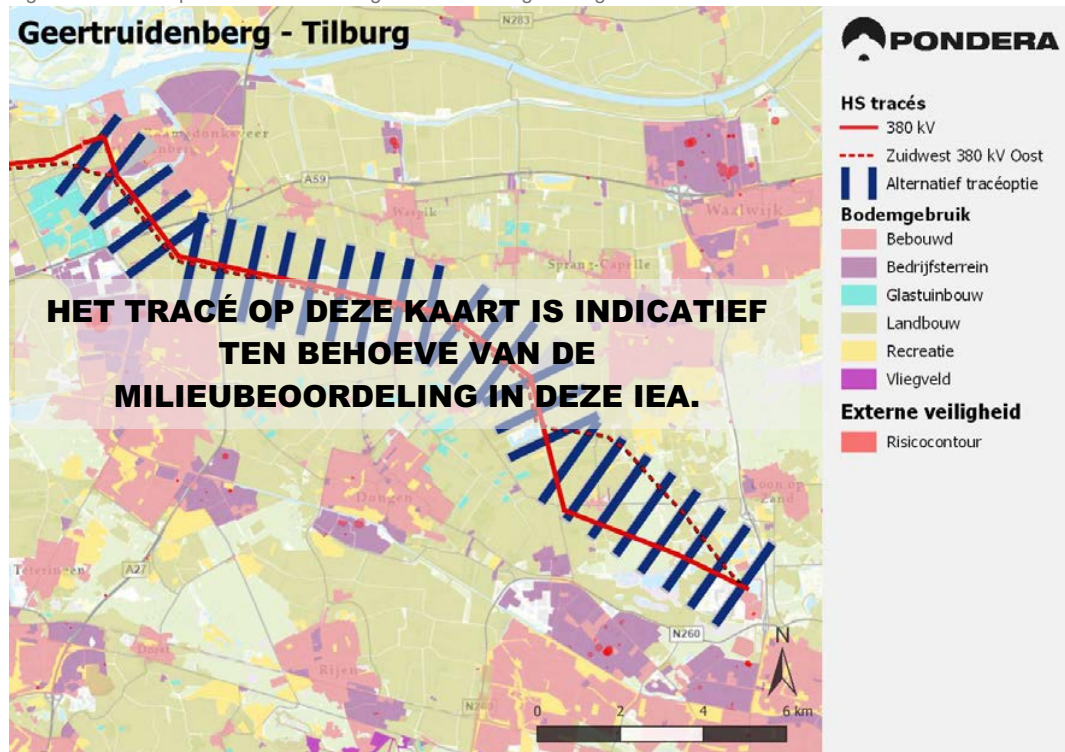
Figuur 30.1 Tracéoptie voor de verbinding Geertruidenberg–Tilburg
