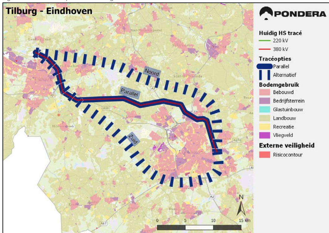
Figuur 40.1 - De tracéopties voor Tilburg–Eindhoven 380kV
