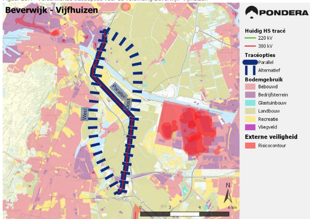
Figuur 26.1 - Verschillende tracéopties voor de verbinding Beverwijk–Vijfhuizen
