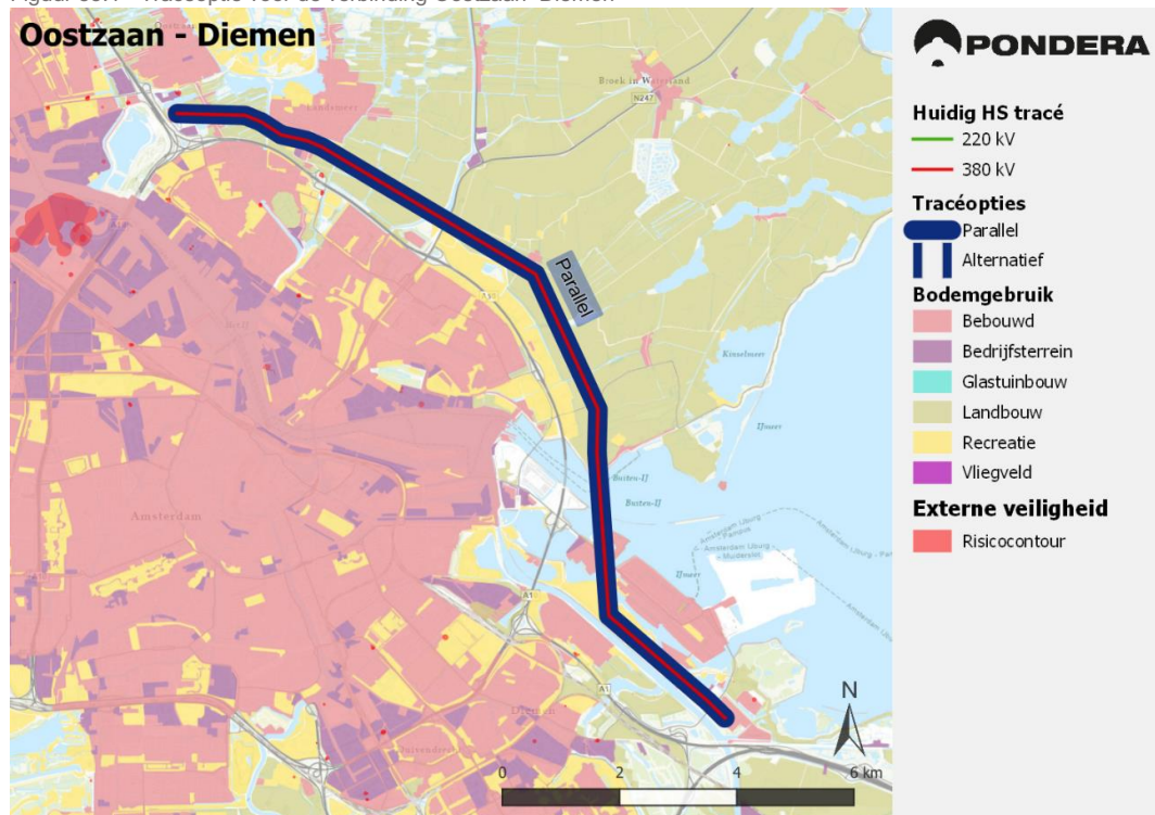
Figuur 35.1 - Tracéoptie voor de verbinding Oostzaan–Diemen
