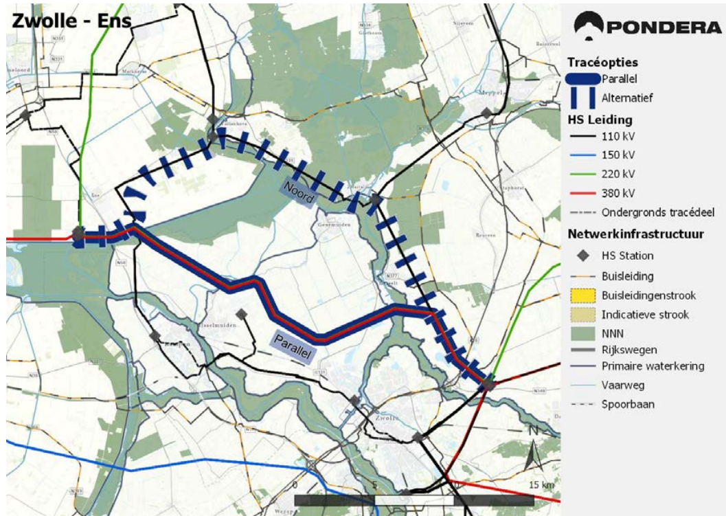
Figuur 2-2 - Tracéopties Zwolle-Ens netwerklaag
