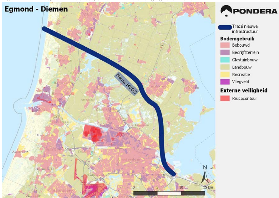
Figuur 42.1 - Tracéoptie voor de ondergrondse HVDC-verbinding Egmond–Diemen
