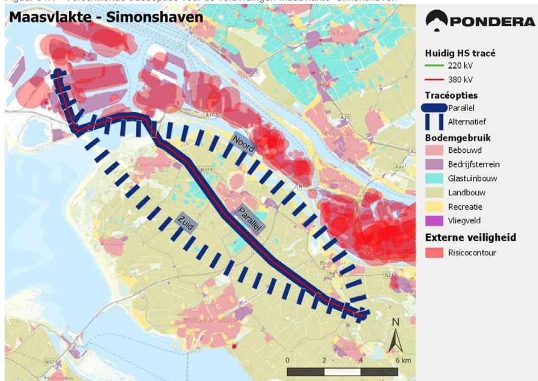
Figuur 34.1 - Verschillende tracéopties voor de verbindingen Maasvlakte–Simonshaven
