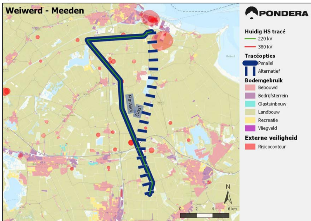
Figuur 41.1 - Tracéopties Weiwerd–Meeden 220kV
