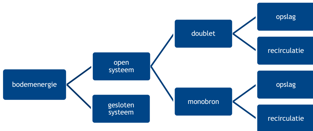
Figuur 3.1 | Overzicht bodemenergiesystemen
