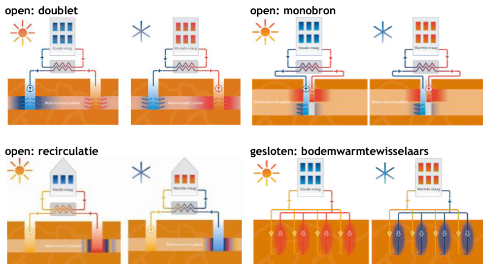
Figuur 3.2 | Schematische weergave verschillende varianten bodemenergie
