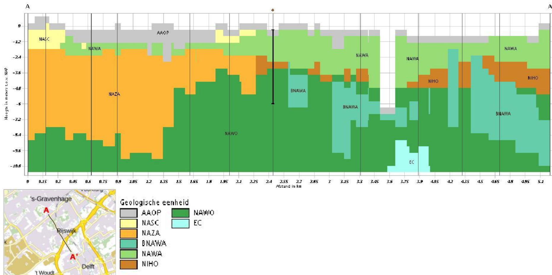
figuur 6: regionale bodemopbouw tracé Prinses Beatrixlaan
