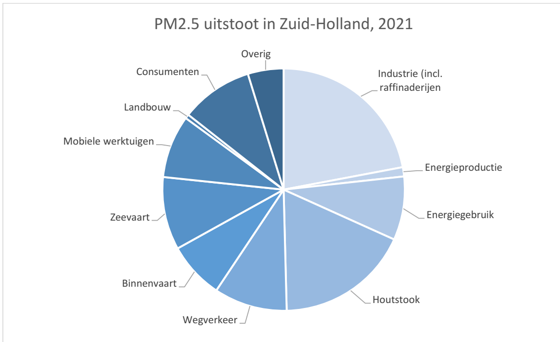
Figuur 14 – Herkomst van de uitstoot van fijn stof PM2,5 in Zuid-Holland in 2021
