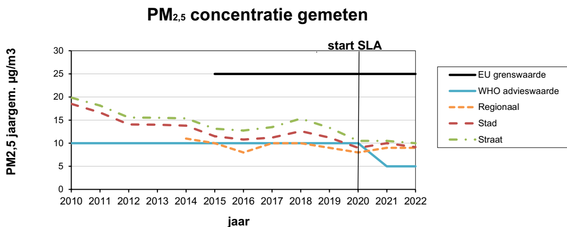
Figuur 9 – trend in gemeten jaargemiddelde concentratie fijn stof fractie PM 2,5 op verschillende typen meetlocaties binnen Zuid-Holland.
