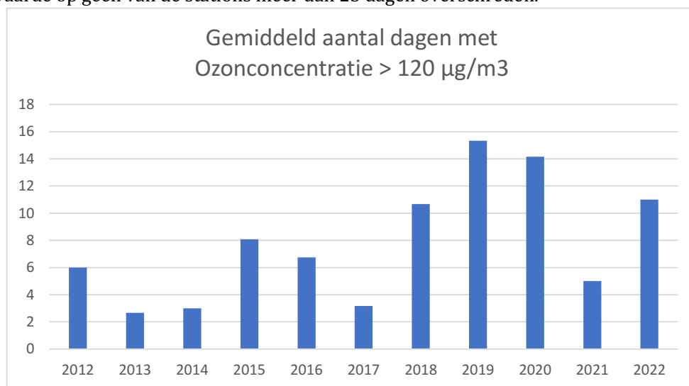
Figuur 10 – trend in het aantal dagen in Zuid-Holland met gemeten Ozonconcentraties groter dan 120 µg/m 3
