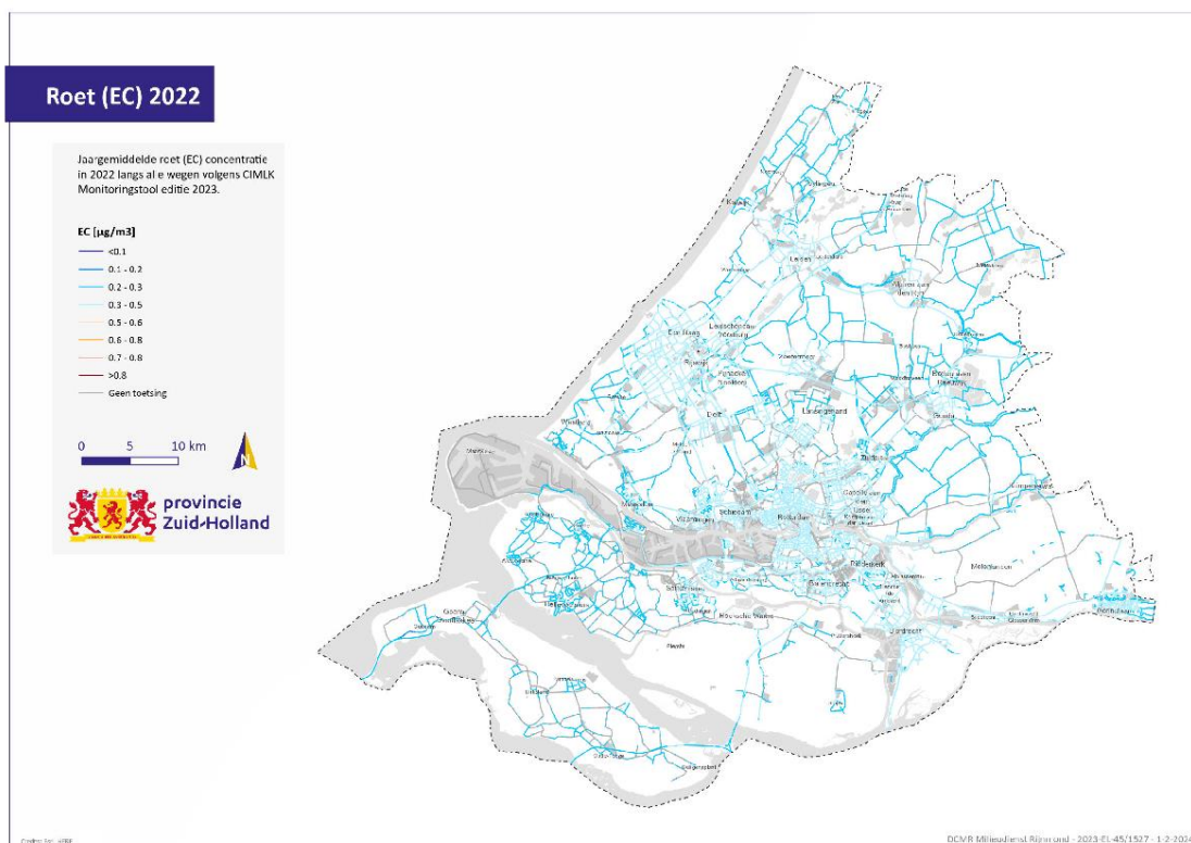
Figuur 6 – jaargemiddelde concentraties roet (EC) langs wegen in Zuid-Holland, 2022
