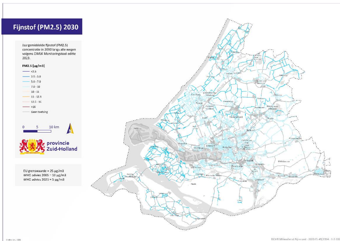
Figuur 17 – Prognose voor concentraties fijn stof (PM2,5) langs wegen in Zuid-Holland, 2030 In aanvulling op de legenda: Voorstel 2022 EU-richtlijn luchtkwaliteit = 10 \mu\text{g}/\text{m}^3 .
