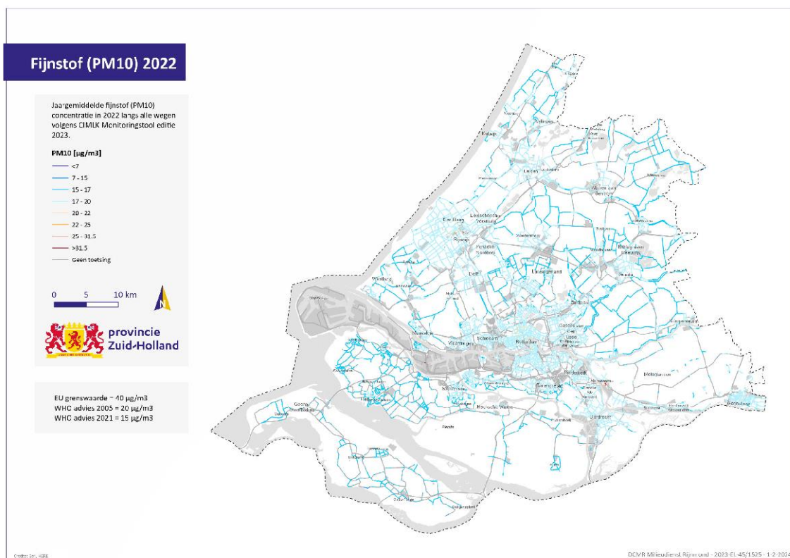
Figuur 4 – Jaargemiddelde concentraties fijn stof (PM10) langs wegen in Zuid-Holland, 2022
