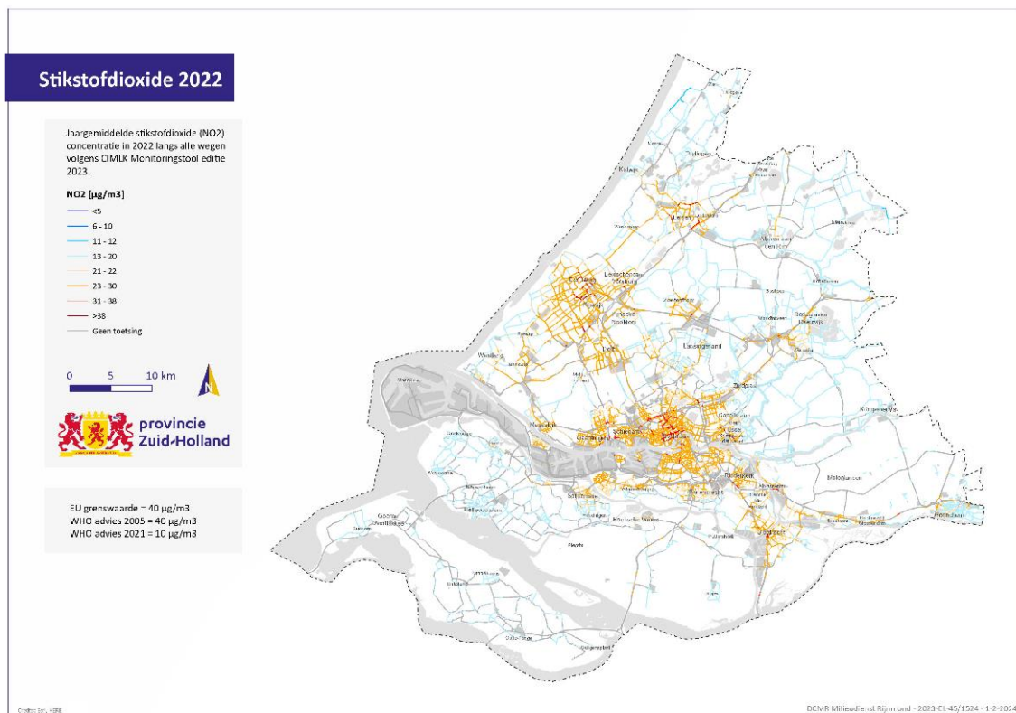
Figuur 3 – Jaarmiddelde concentraties stikstofdioxide (NO 2 ) langs wegen in Zuid-Holland, 2022
