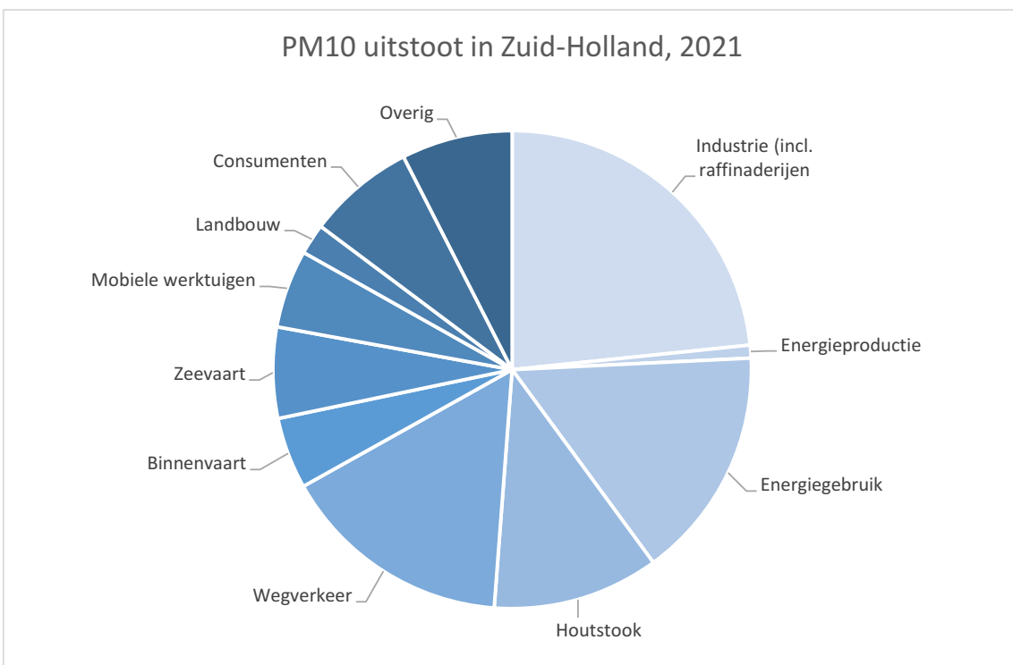
Figuur 13 – Herkomst van de uitstoot van fijn stof PM10 in Zuid-Holland in 2021
