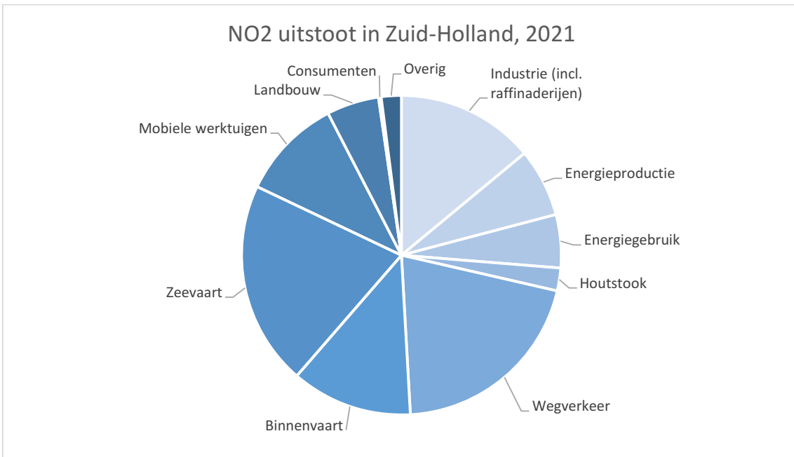
Figuur 12 – Herkomst van de uitstoot van stikstofoxiden in Zuid-Holland in 2021
