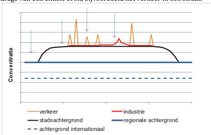
Figuur I - Dwarsdoorsnede van het werkgebied met de denkbare opbouw van concentraties van luchtvervuiling en de verschillende herkomst van de concentratiebijdragen. De pijlen geven de plaats van de verschillende typen meetpunten weer.
