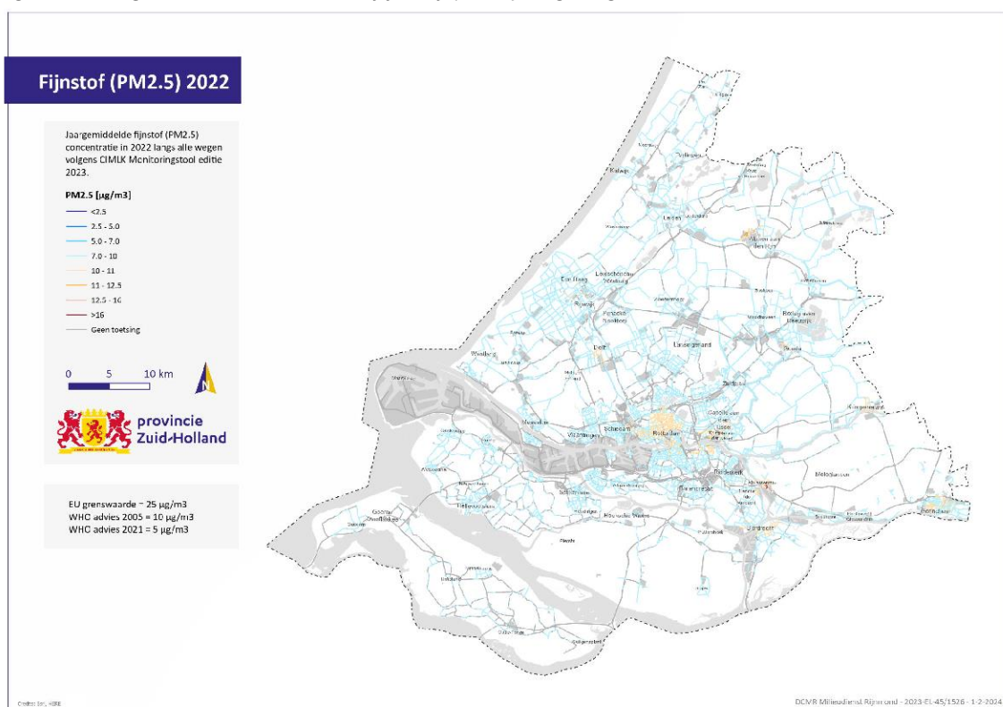
Figuur 5 – Jaargemiddelde concentraties fijn stof (PM2.5) langs wegen in Zuid-Holland, 2022
