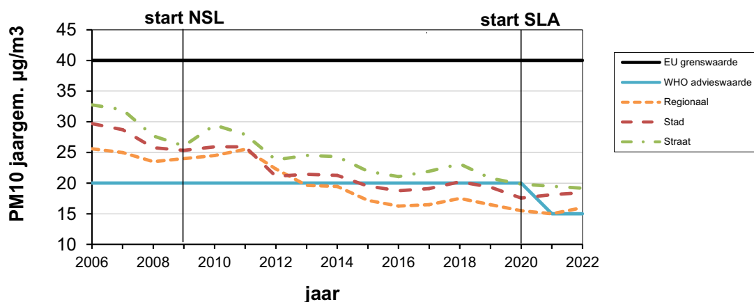
Figuur 8 - trend in gemeten jaargemiddelde concentratie fijn stof fractie PM 10 op verschillende typen meetlocaties binnen Zuid-Holland.
