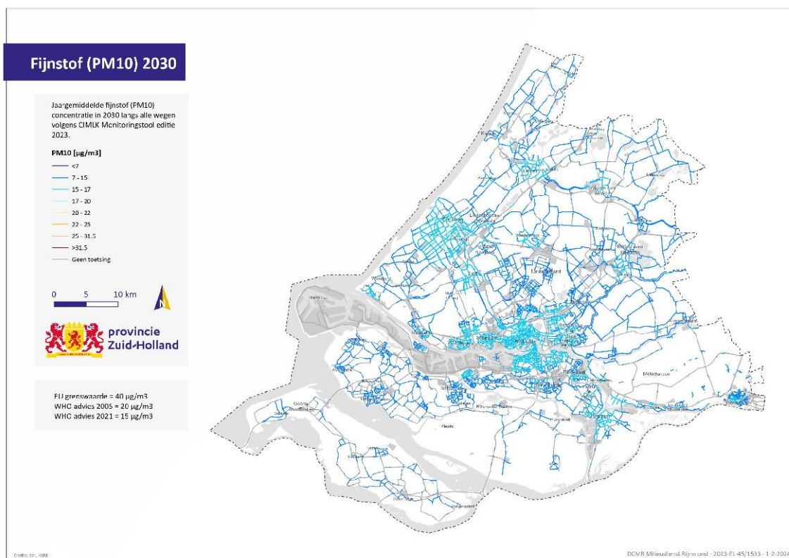
Figuur 16 – Prognose voor concentraties fijn stof (PM10) langs wegen in Zuid-Holland, 2030 In aanvulling op de legenda: Voorstel 2022 EU-richtlijn luchtkwaliteit = 20 \mu\text{g}/\text{m}^3 .
