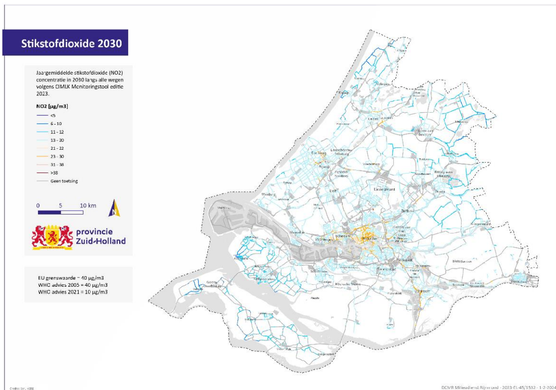
Figuur 15 – Prognose voor concentraties stikstofdioxide (NO 2 ) langs wegen in Zuid-Holland, 2030. In aanvulling op de legenda: Voorstel 2022 EU-richtlijn luchtkwaliteit = 20 \mu\text{g}/\text{m}^3 .
