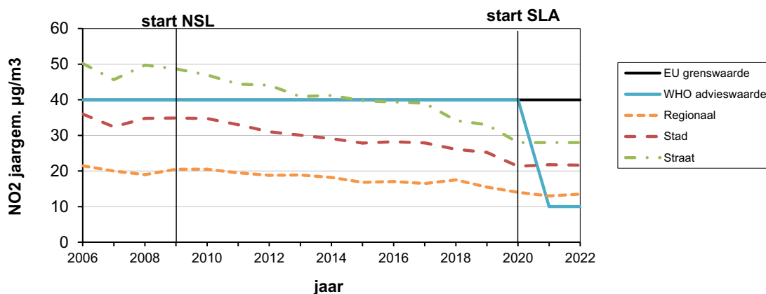
Figuur 7- trend in gemeten jaargemiddelde concentratie stikstof op verschillende typen meetlocaties binnen Zuid-Holland.
